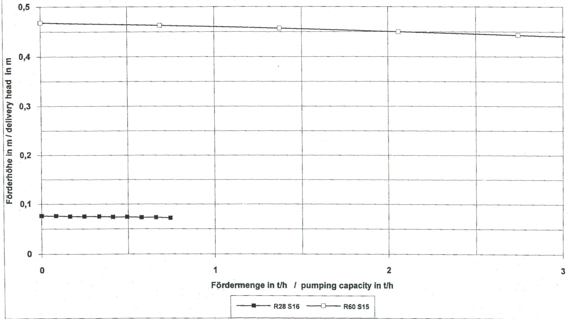
Kennlinien der EM - Pumpen / characteristics of em - pumps Zinn 450 °C / tin 450 °C
