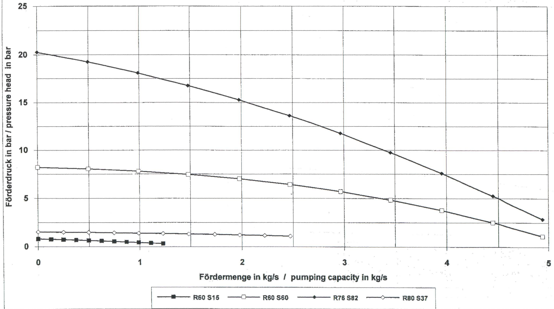
Kennlinien der EM - Pumpen / characteristics of em - pumps Natrium 250 °C / sodium 250 °C
