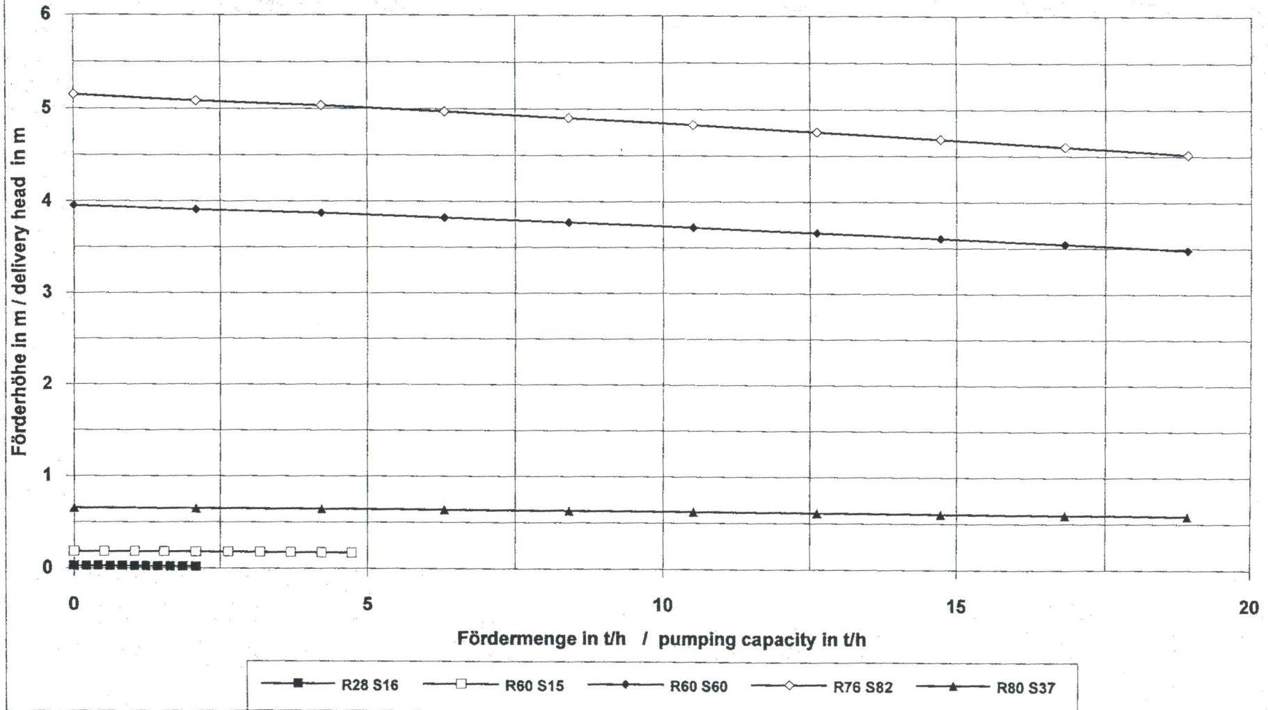
Kennlinien der EM - Pumpen / characteristics of em - pumps Blei 450 °C / lead 450 °C
