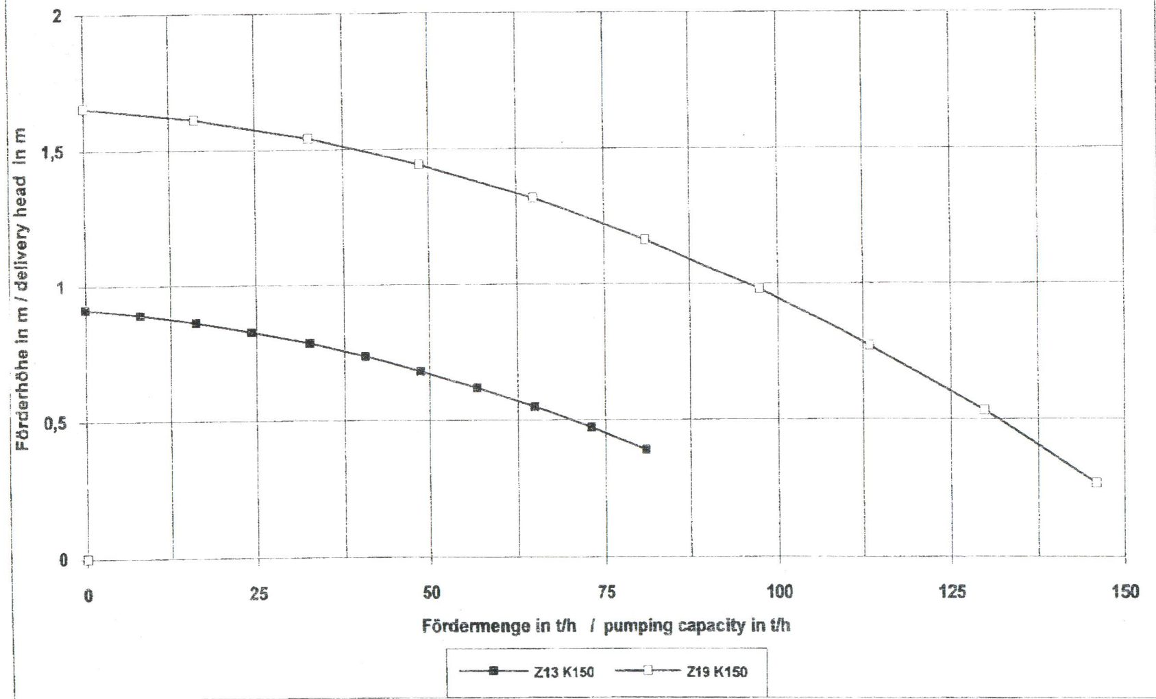
Kennlinien der EM - Pumpen / characteristics of em - pumps Zink 500 °C / zinc 500 °C
